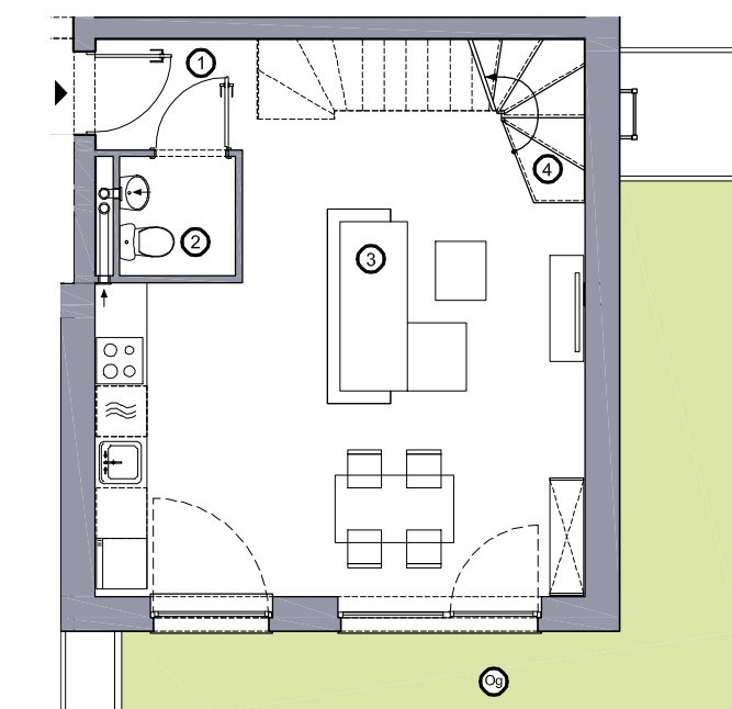
Rzut parteru
