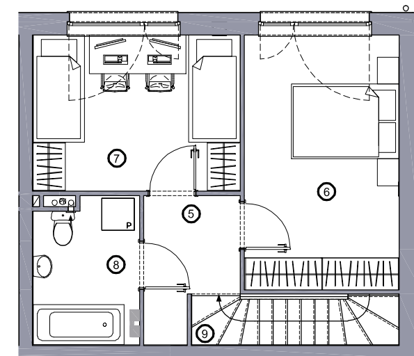
Rzut 1 piętra
