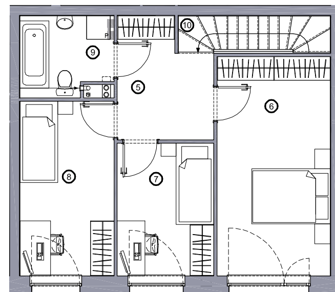
Rzut 1 piętra
