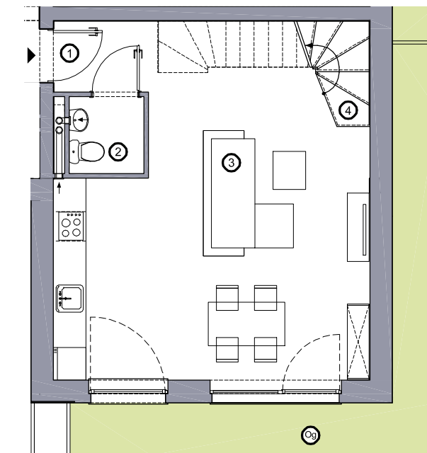
Rzut parteru
