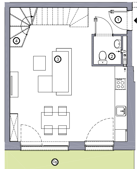
Rzut parteru
