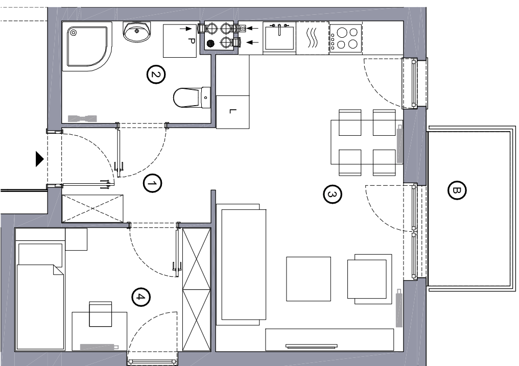
RZUT MIESZKANIA
